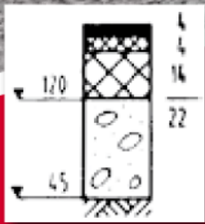
Bitumendecke
